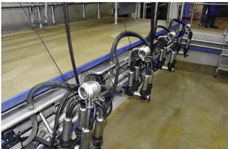
Komfort für Kuh und Melker: Das robuste Melkzeug MC73 aus Edelstahl mit der innovativen TF (Top Flow) Technologie ermöglicht einen schnellen und ungestörten Milchfluss aus dem Sammelstück.
