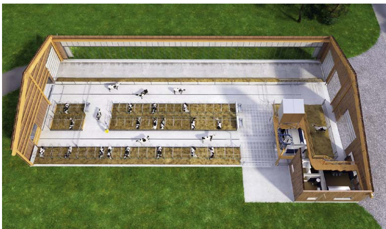
Sicht von oben: Der schlüsselfertige Normroboterstall VMS für 70 Kühe
